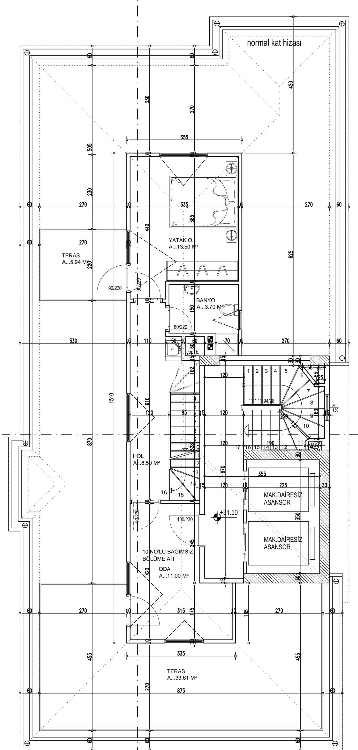
ÇATI ARASI KAT PLANI
